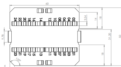
Fig. 5 Vista superior contenedor
