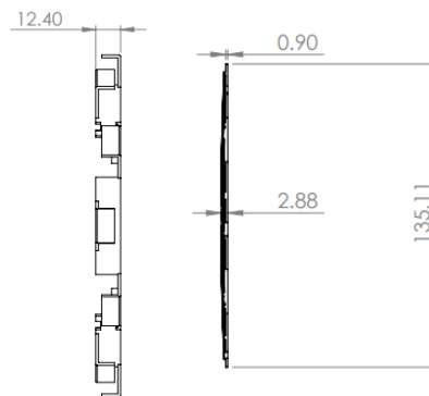
Fig. 4 Vista lateral charola, cubierta
