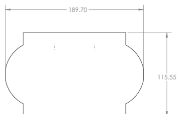
Fig. 3 Vista frontal charola
