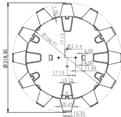
Fig. 1 Vista superior charola
