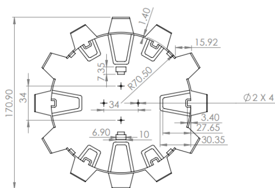
Fig. 1 Vista superior charola
