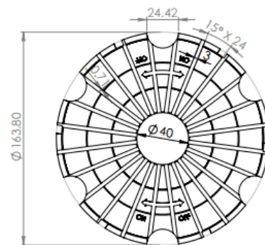
Fig. 2 Vista superior cubierta
