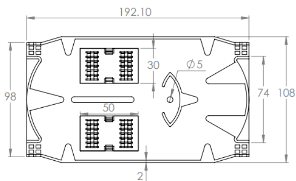
Fig. 1 Vista superior charola
