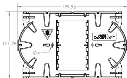
Fig. 1 Vista superior charola
