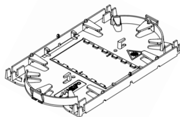
Fig. 2 Vista isométrica charola
