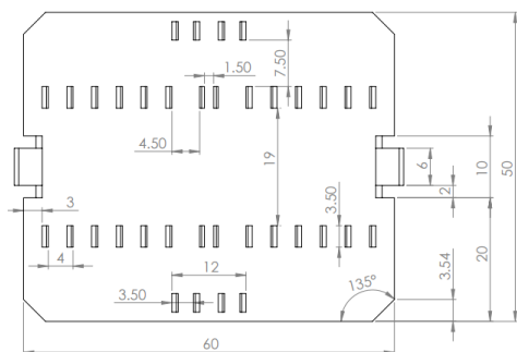
Fig. 3 Vista superior contenedor
