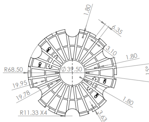
Fig. 2 Vista superior cubierta
