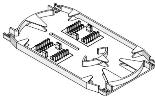
Fig. 2 Vista isometrica charola
