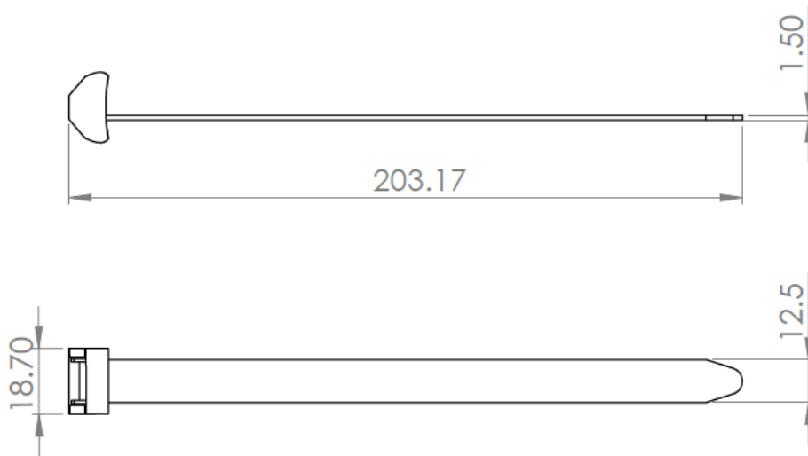
Fig.1 Cuerpo de cincho atacable CT-203
