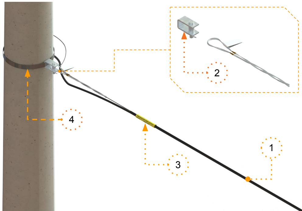
Fig. 1: Ejemplo de instalación de un cable F8 con los preformados para mensajero de acero
