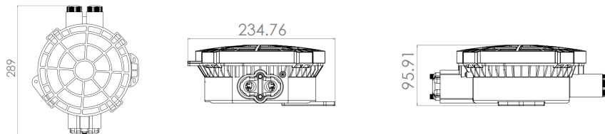
Fig 1 Dimensiones generales del producto establecidas en mm.
