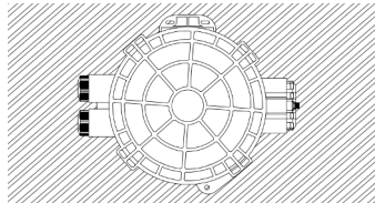
Fig 3 Instalación Enterrada
