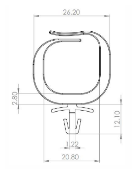
Fig. 2 Vista frontal
