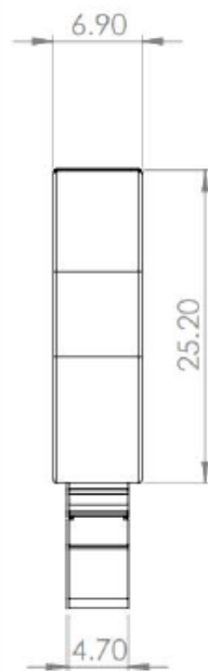
Fig. 3 Vista lateral
