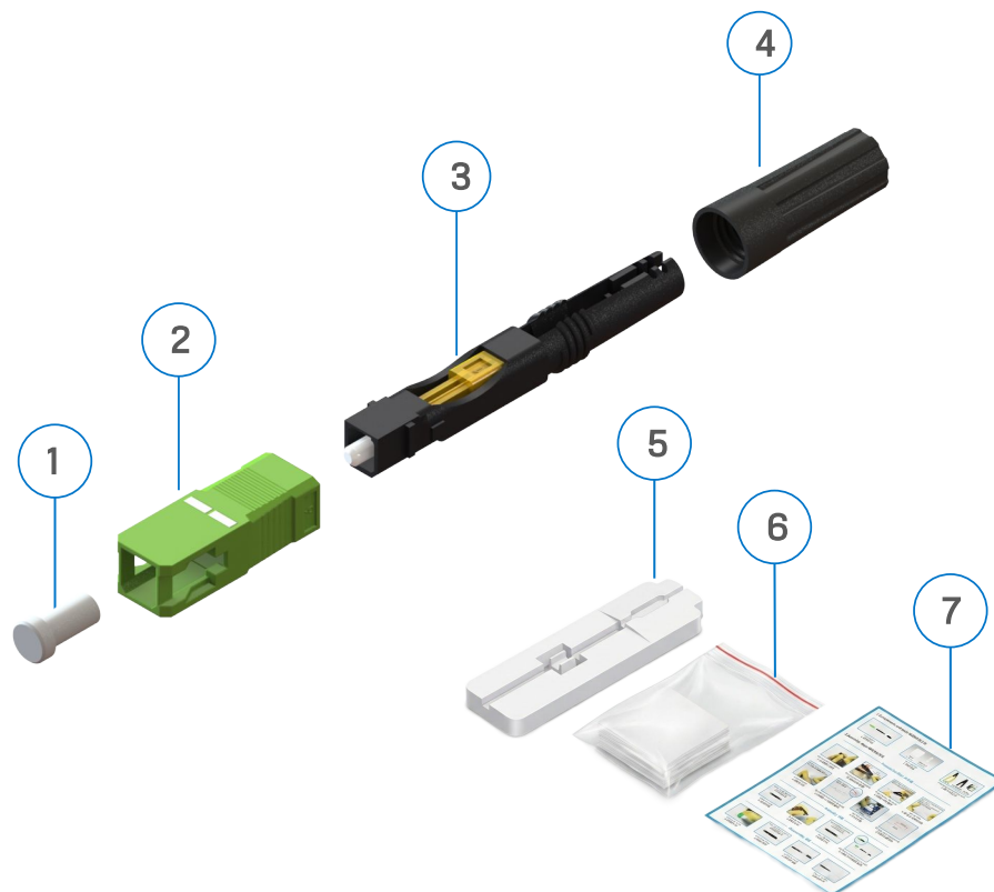
Fig. 2 Componentes y accesorios del conector
