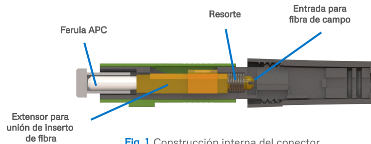
Fig. 1 Construcción interna del conector
