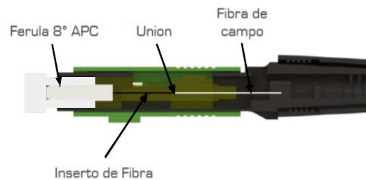
Fig. 1 Construcción interna del conector
