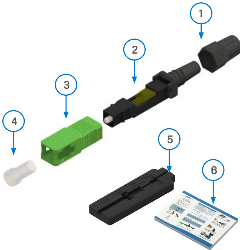
Fig. 2 Componentes y accesorios del conector
