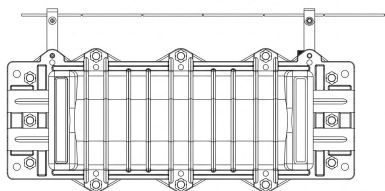
Fig. 1 Instalación aérea
