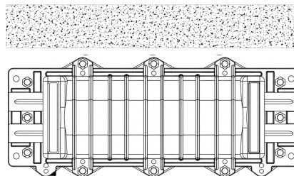
Fig. 2 Instalación subterránea
