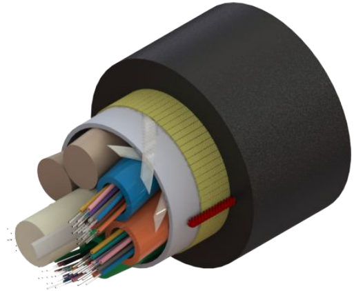
VISTA ISOMÉTRICA / FOSPC-048-F-ADSSJ2E
