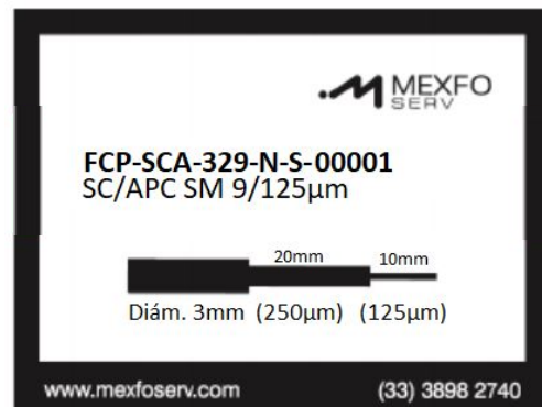
Fig 3. Diseño de la ayuda visual en la bolsa individual
