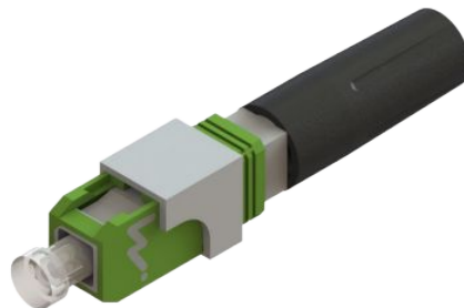
Fig.1 Imagen isométrica del conector prepulido
