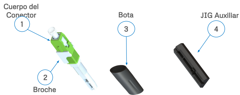
Fig 2. Componentes del conector prepulido
